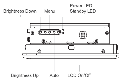
Right I/O
