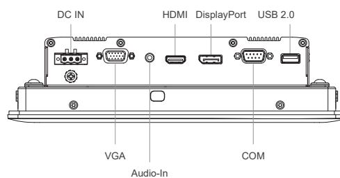
Right I/O
