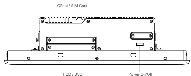
Right I/O
