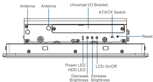
Left I/O
