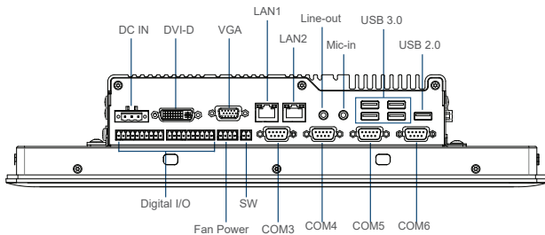
Left I/O
