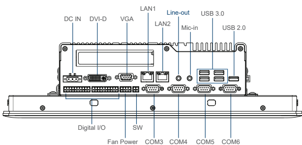
Left I/O
