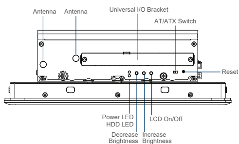
Left I/O
