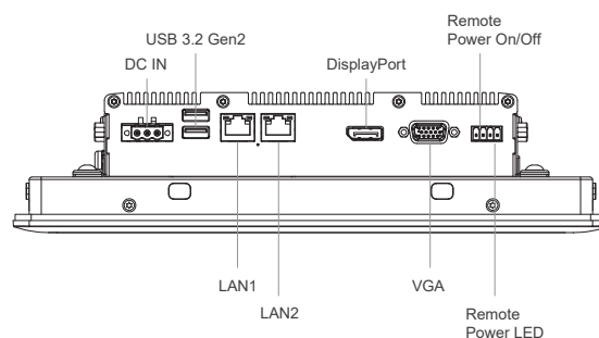
Right I/O
