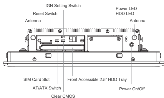
Left I/O
