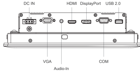
Right I/O
