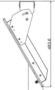
STAND ANGLE
