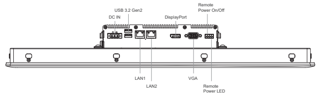
Right I/O
