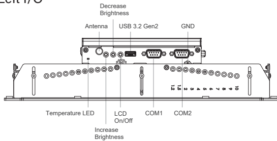
Left I/O
