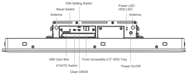
Left I/O
