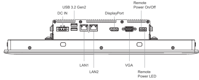
Right I/O
