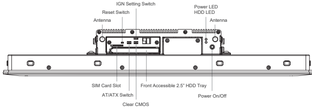
Left I/O
