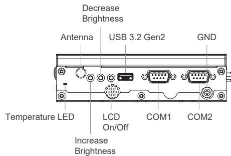
Left I/O
