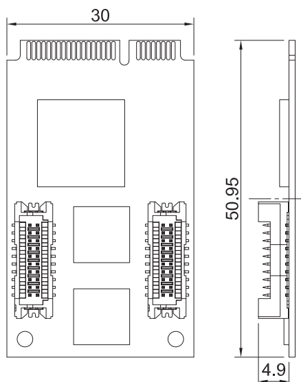
Mini PCIe Card
