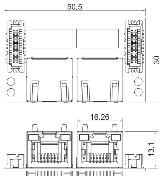
LAN I/O Card
