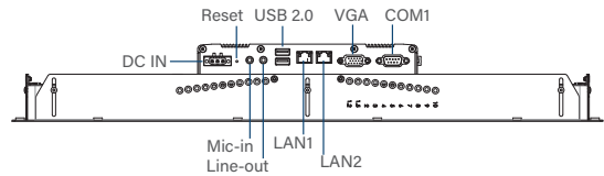
Right I/O
