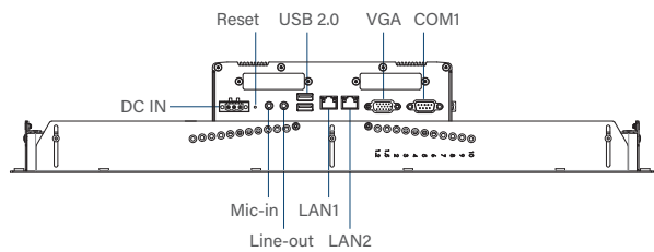
Right I/O
