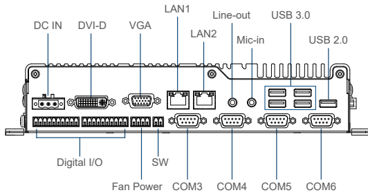
Left I/O
