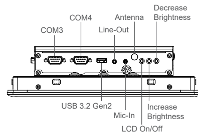
Right I/O
