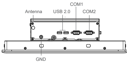
Left I/O
