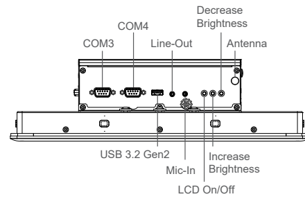
Right I/O
