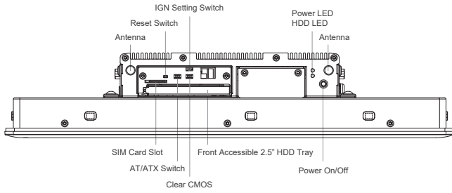
Left I/O
