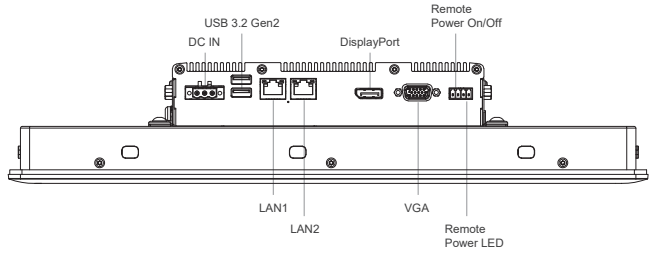
Right I/O
