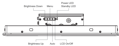
Right I/O
