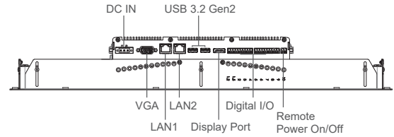
Right I/O
