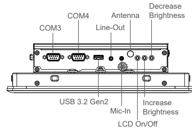
Right I/O
