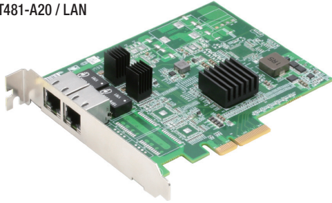
PER-T481-A20 / LAN
